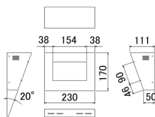
外形寸法図
