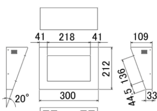
外形寸法図
