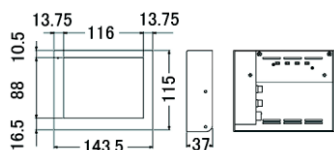
壁掛け金具未装着
