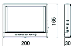
外形寸法図
