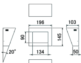
外形寸法図
