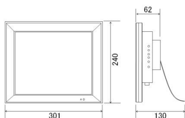
外形寸法図
