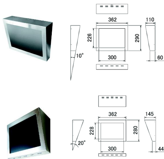
外形寸法図
