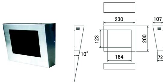
外形寸法図
