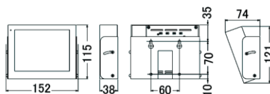
角度調整付き壁掛け金具装着
