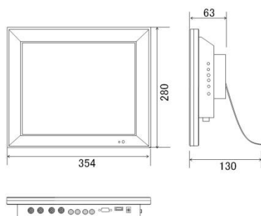
コネクタ図
