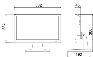
外形寸法図
