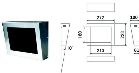
外形寸法図
