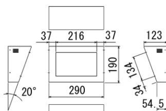
外形寸法図
