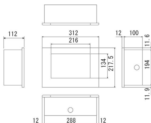
外形寸法図
