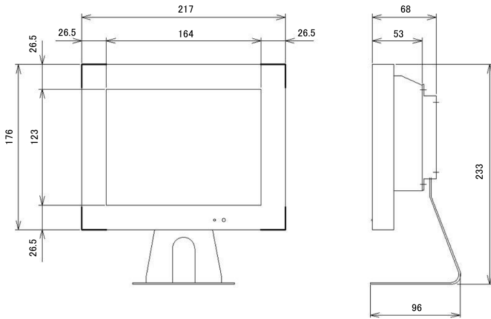
外形寸法図/NM-LCDW80HVS
